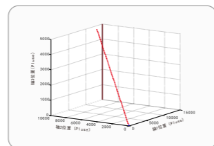
空间直线插补轨迹曲线
