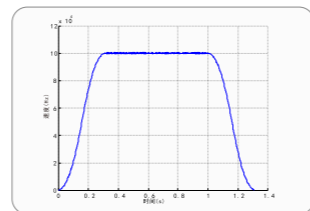
圆弧插补合速度曲线
