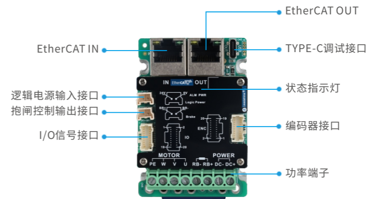
(LD3M-EC驱动器接口说明)
