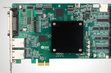
DMC-E5064S-AxxP04-PCIe运动控制卡配置方案
