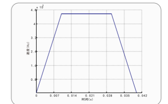
对称T型速度曲线
