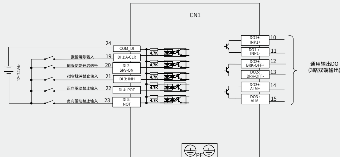
速度/力矩控制接线图
