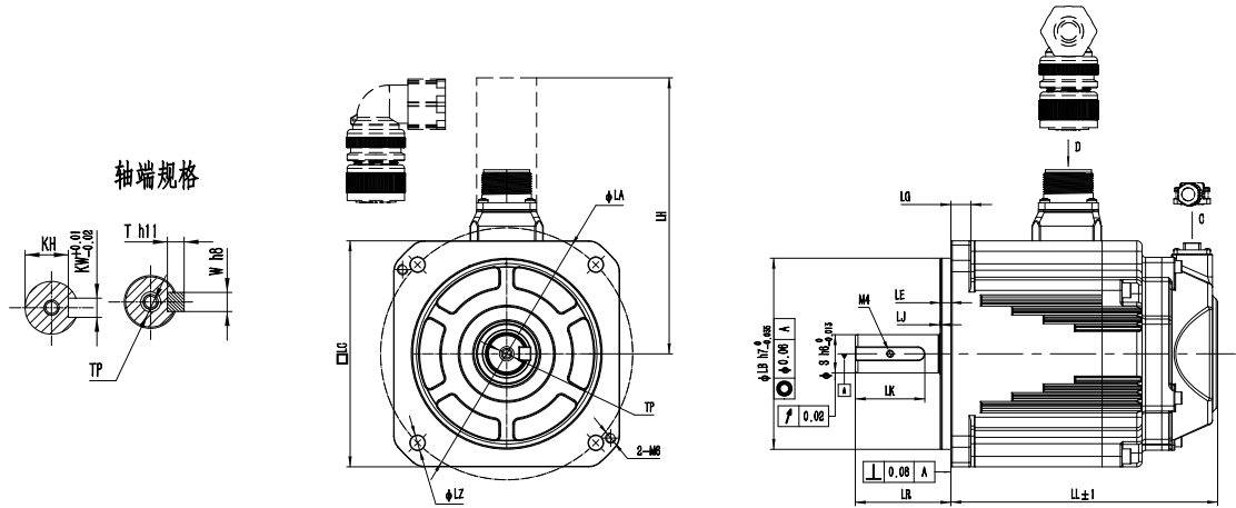
M5-130机座
