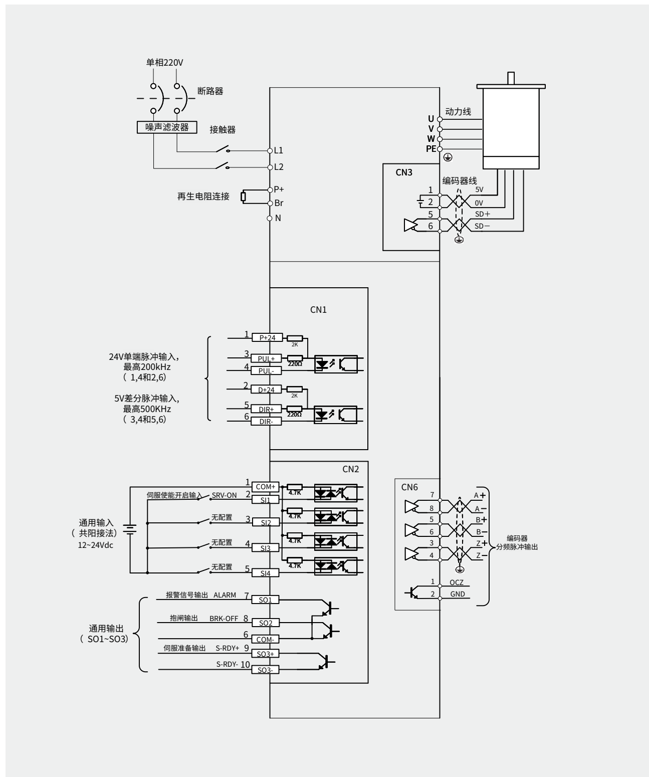
■ 驱动器接线图
