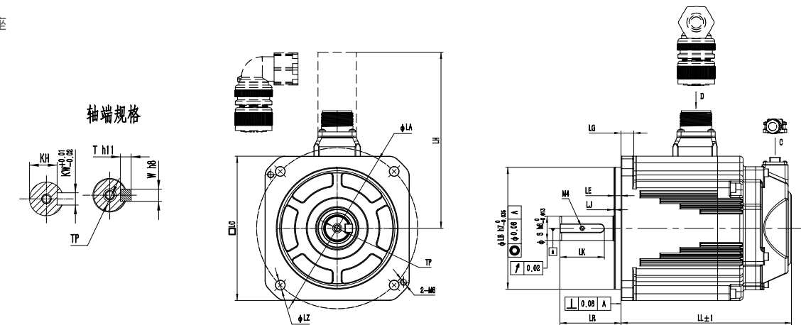
M6-130机座
