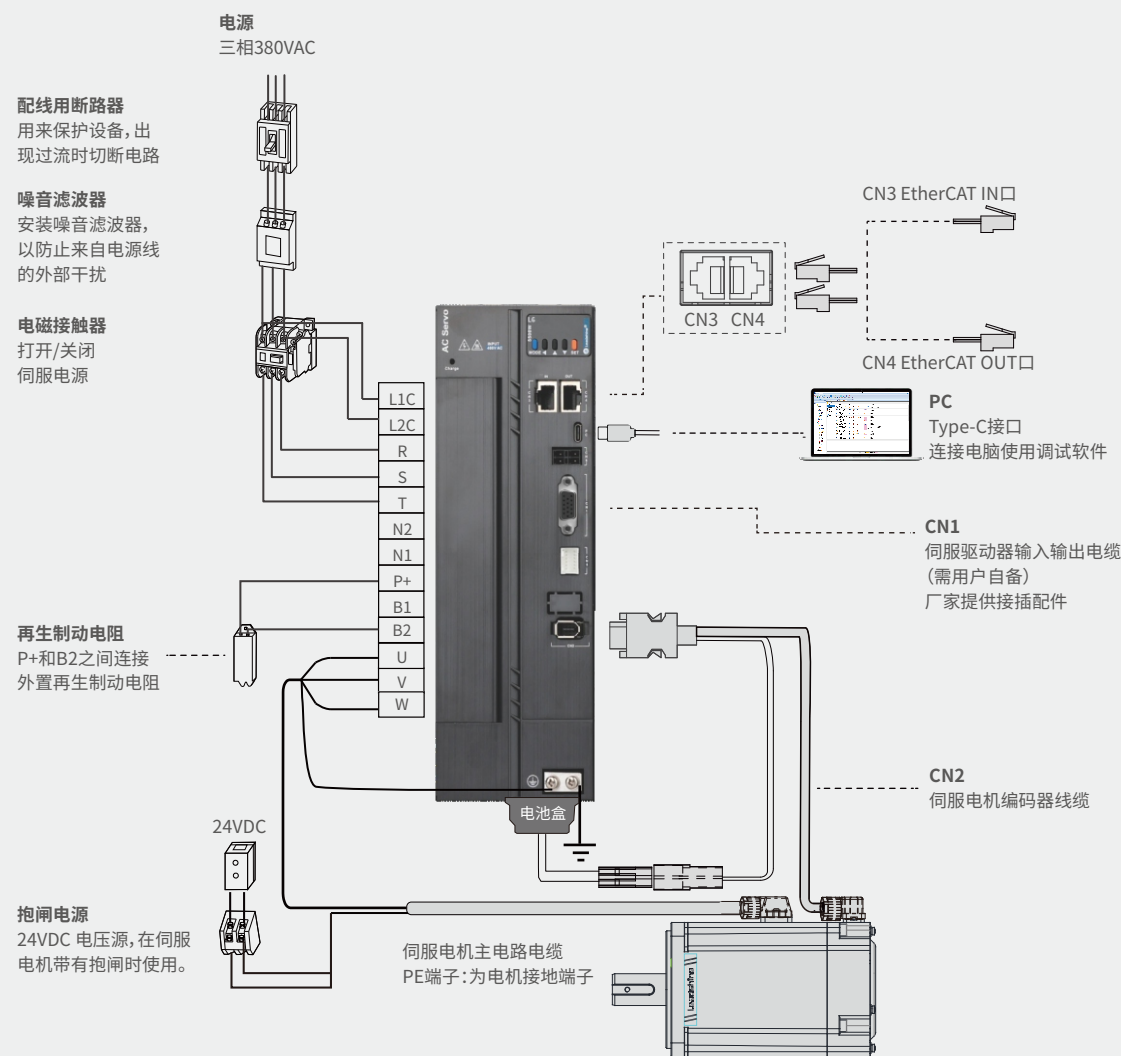
L6N-4400T~7500T外围设备连接图
