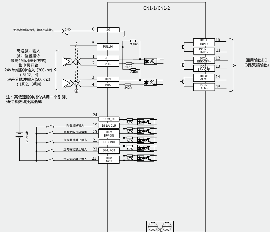
位置控制模式接线
