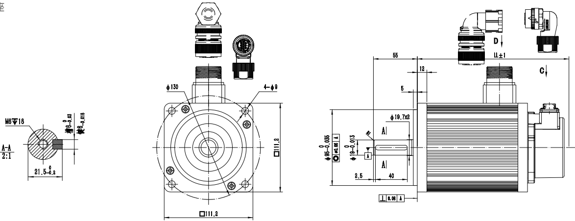
M6-110机座
